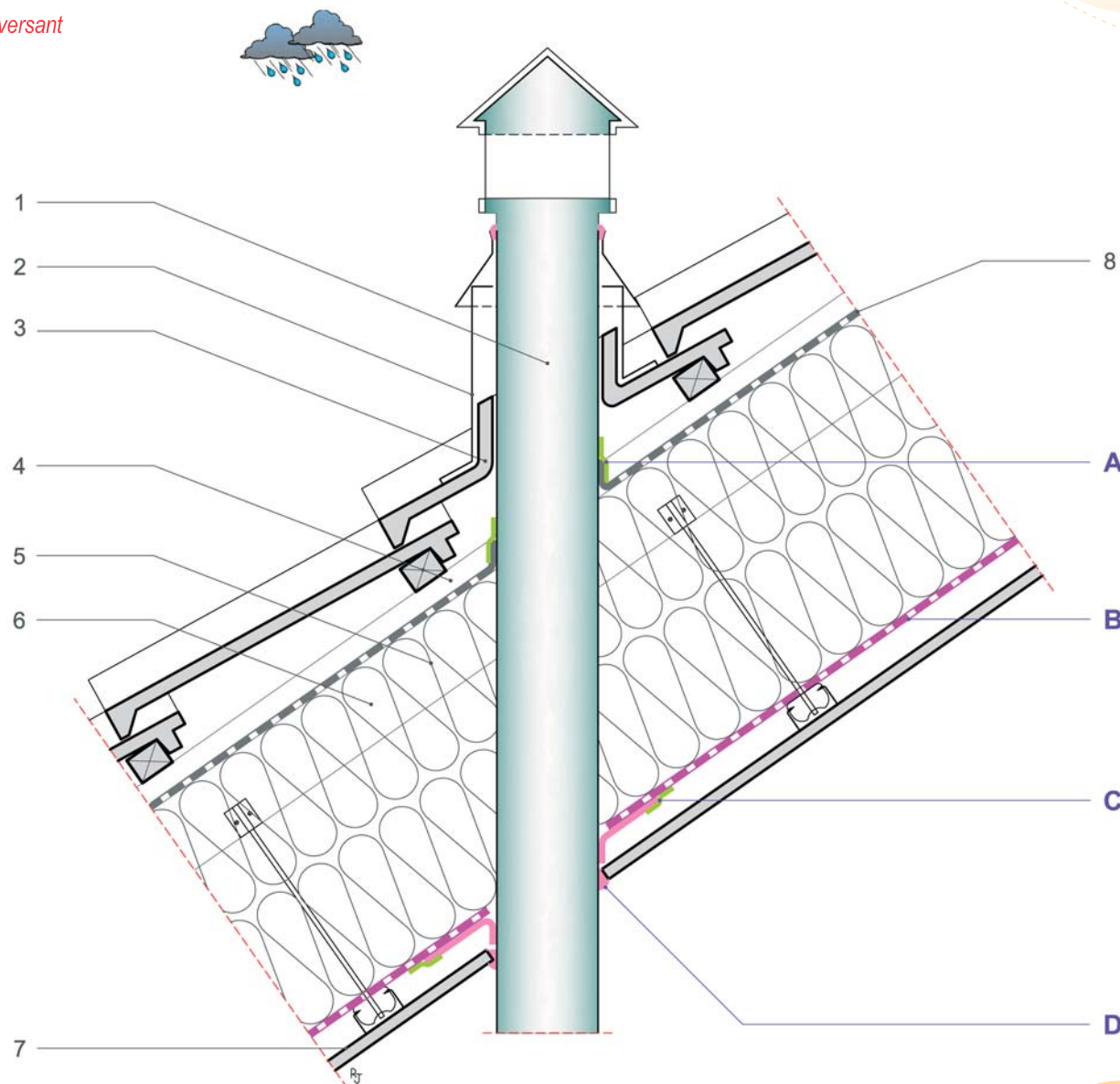
Coupe verticale
