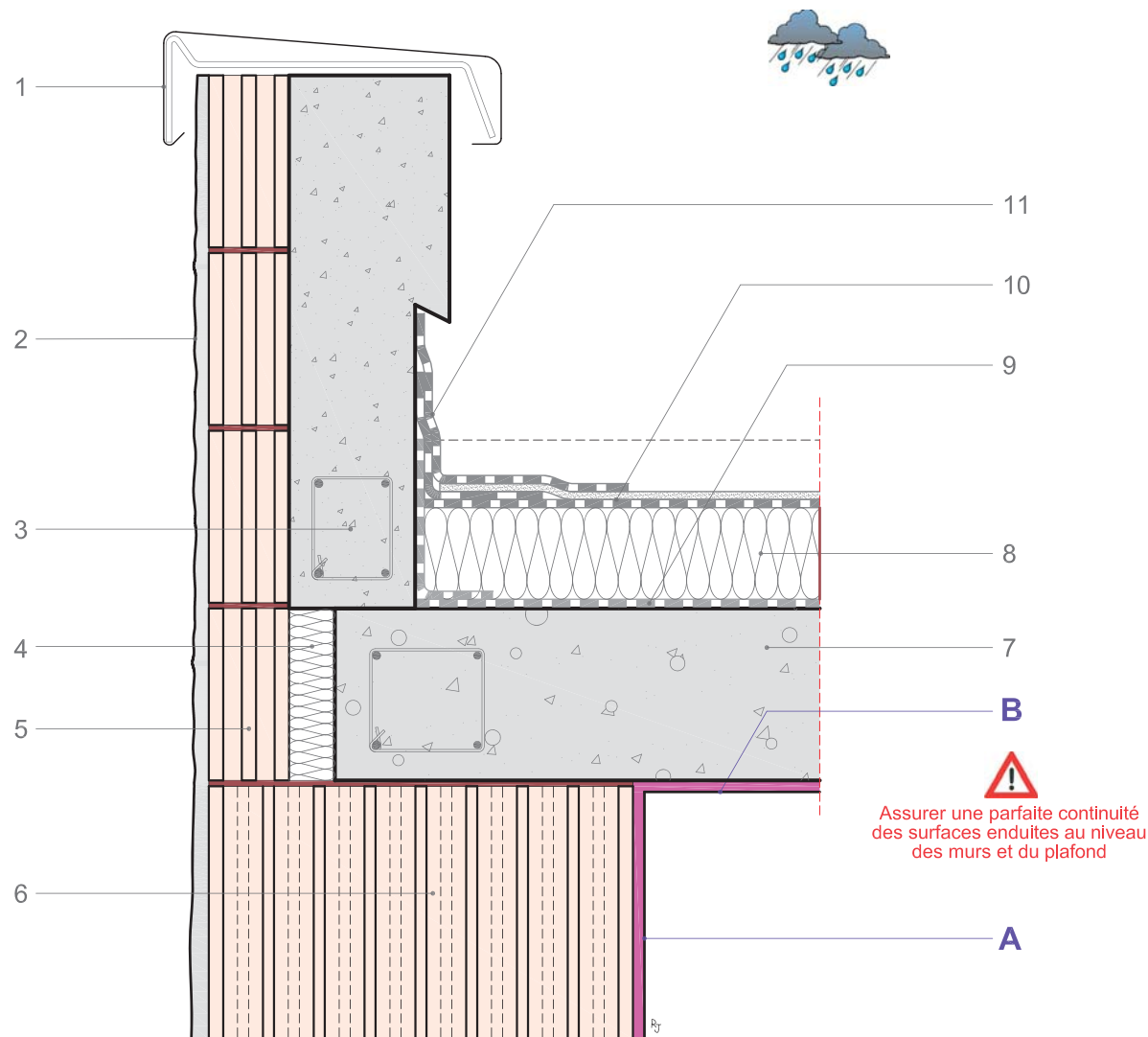
Coupe verticale
