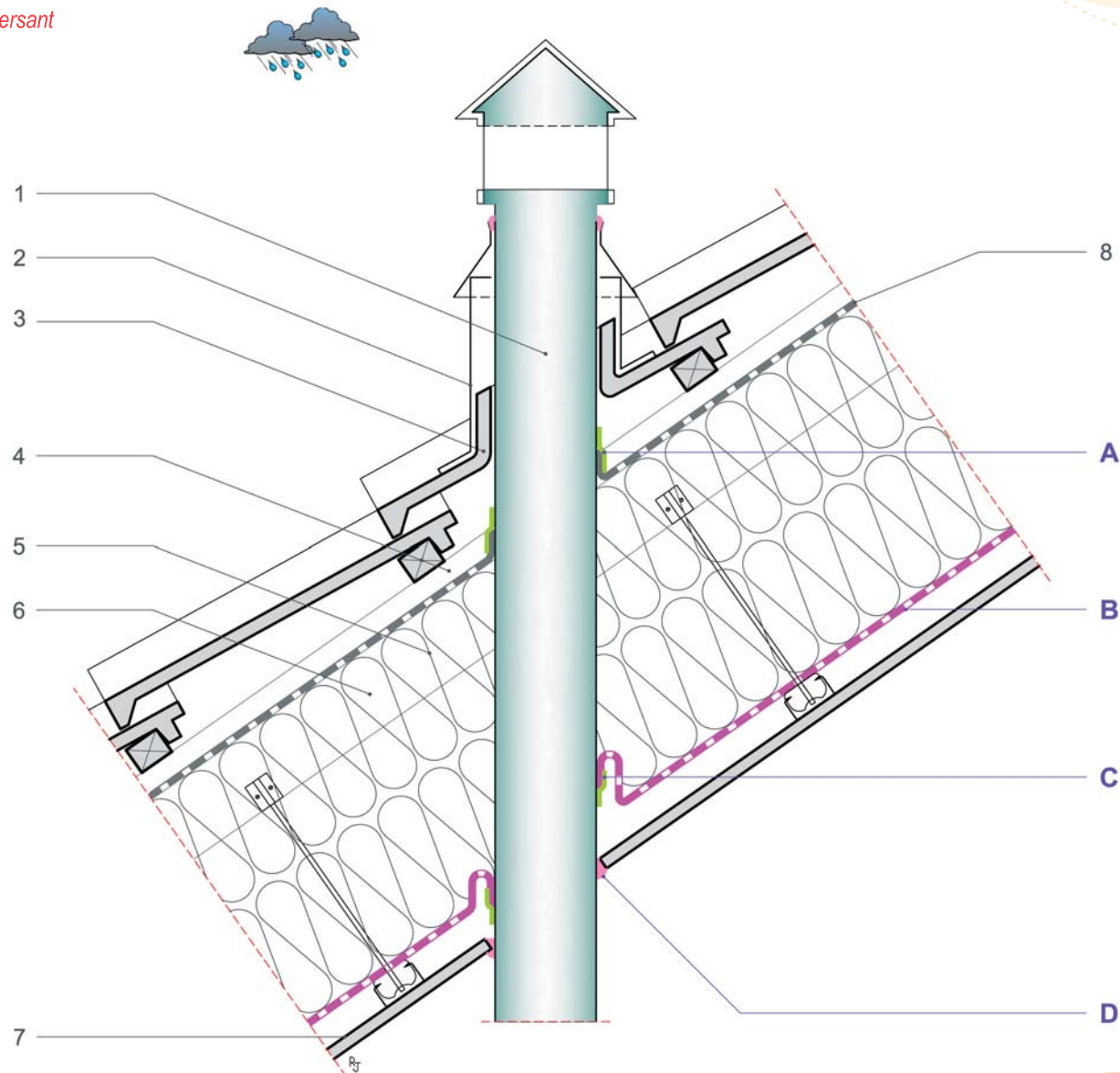
Coupe verticale
