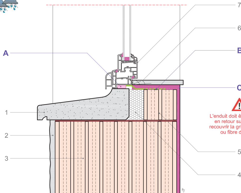
Coupe verticale
