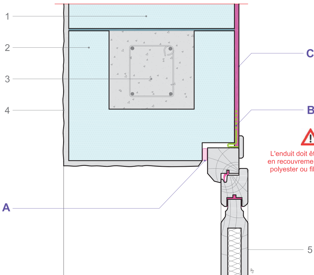
Coupe verticale
