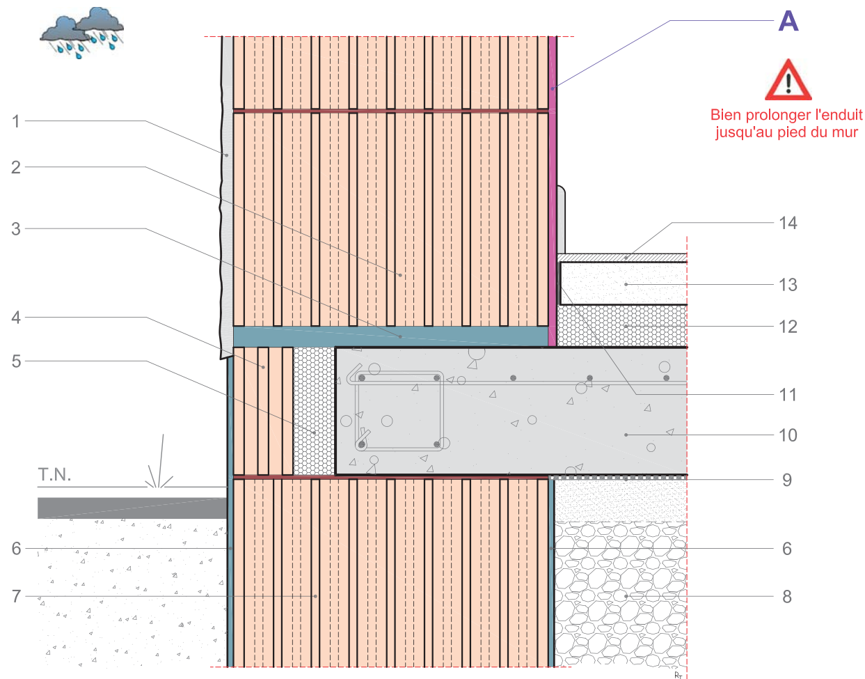
Coupe verticale
