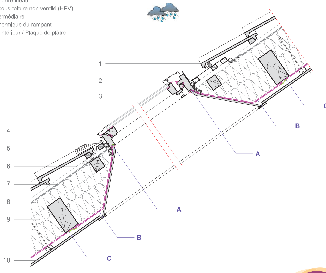
Coupe verticale
