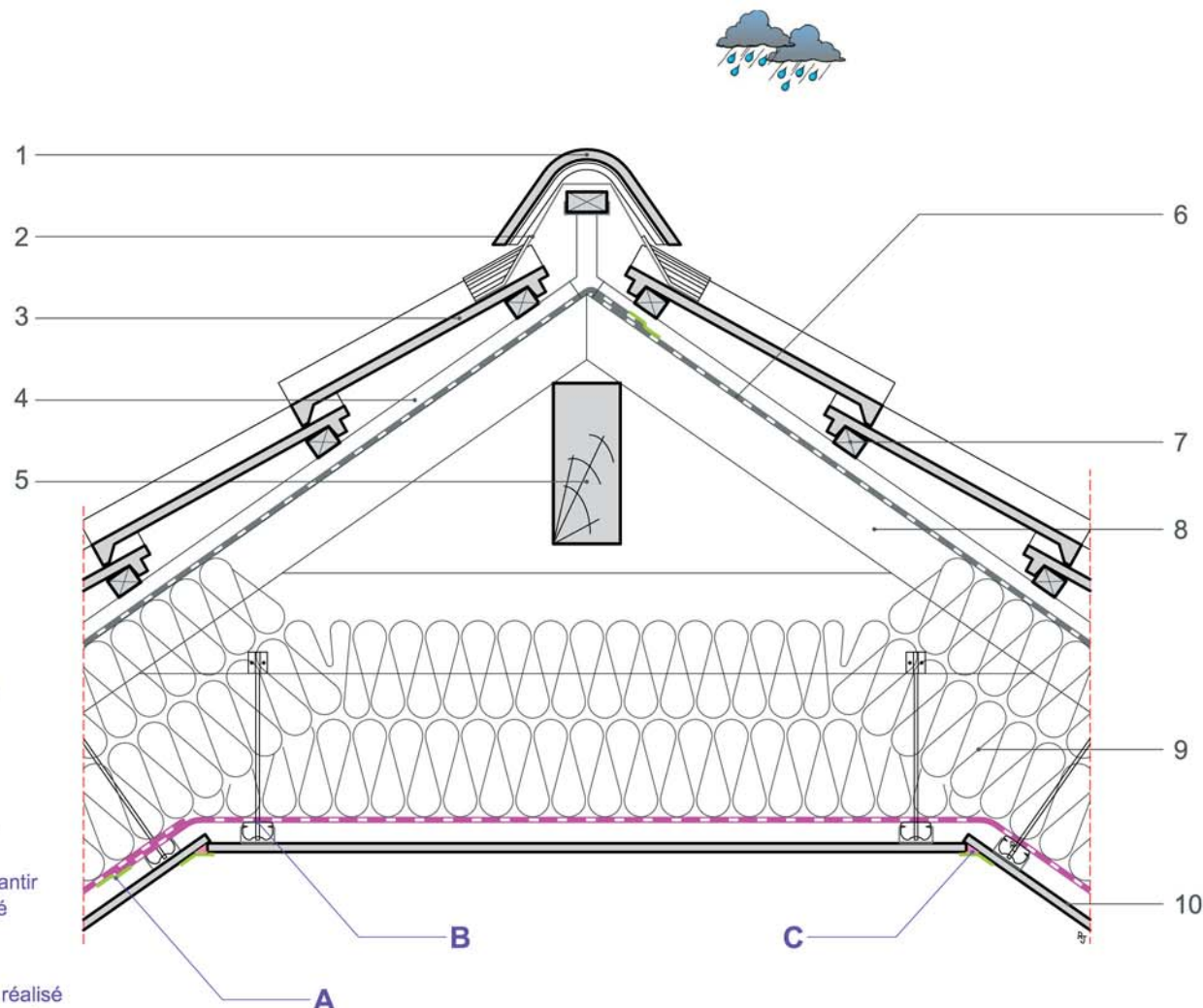
Coupe verticale
