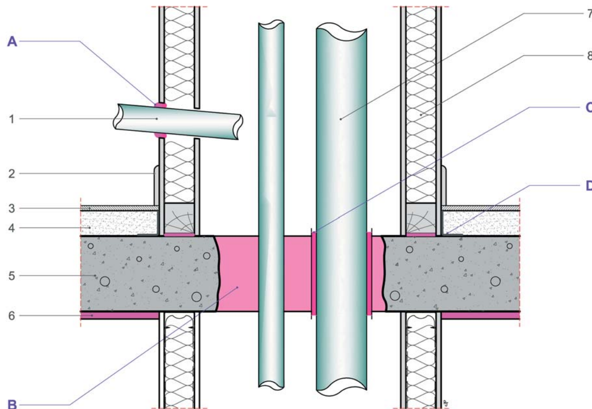
Coupe verticale
