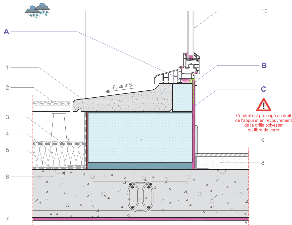
Coupe verticale
