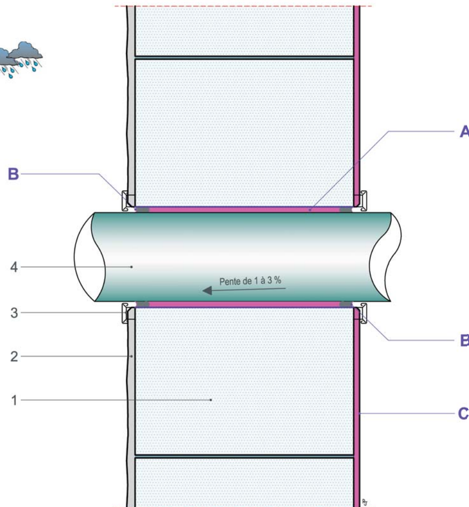
Coupe verticale
