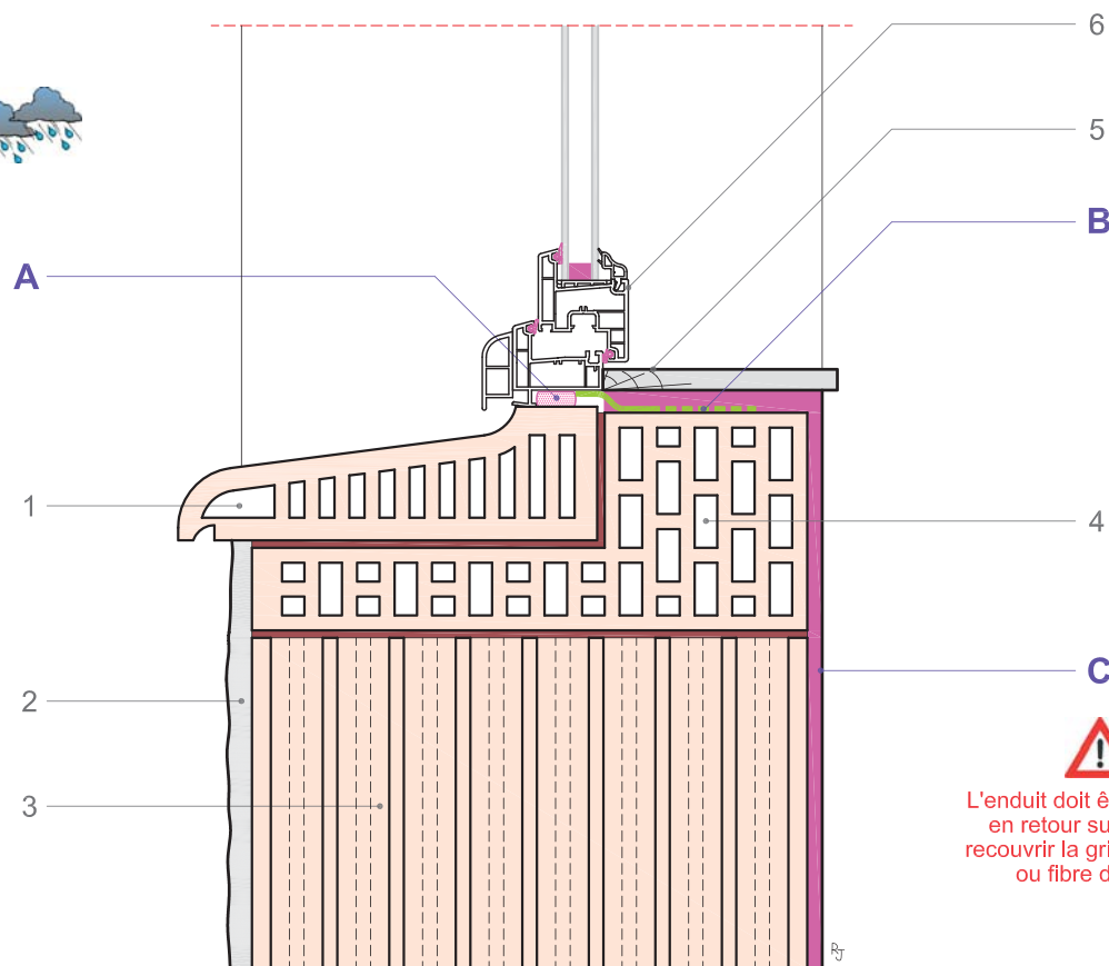
Coupe verticale
