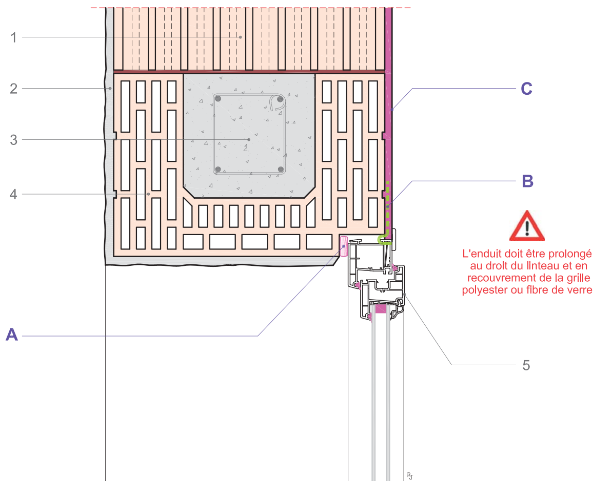
Coupe verticale
