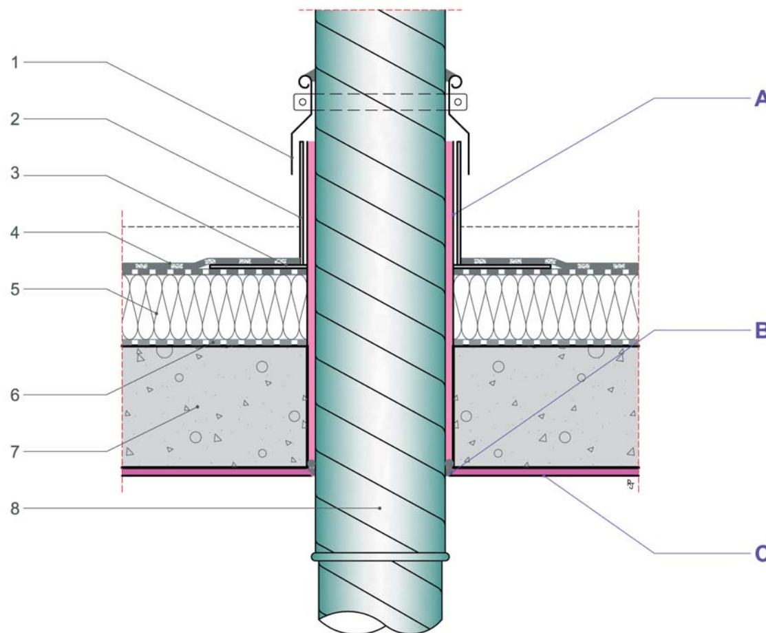
Coupe verticale
