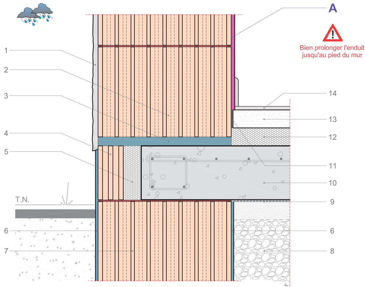
Coupe verticale
