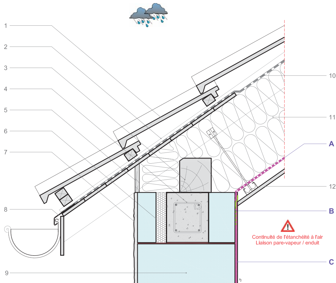
Coupe verticale
