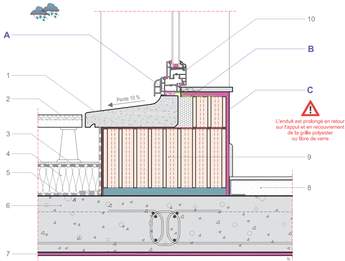
Coupe verticale
