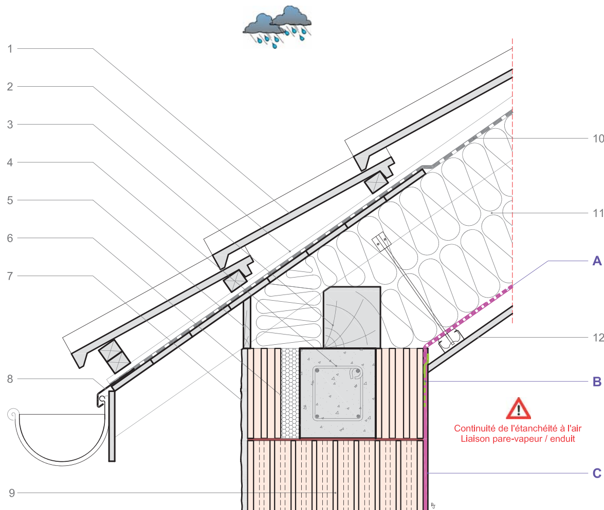
Coupe verticale
