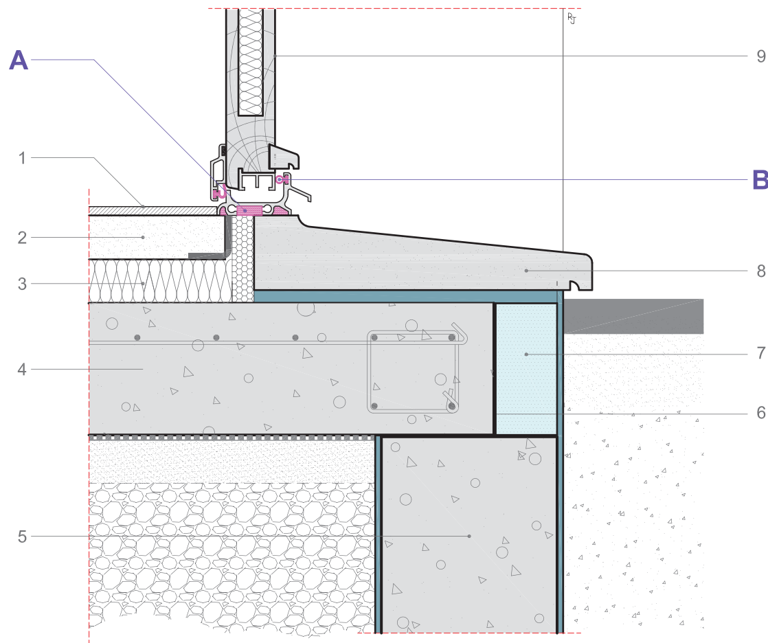
Coupe verticale
